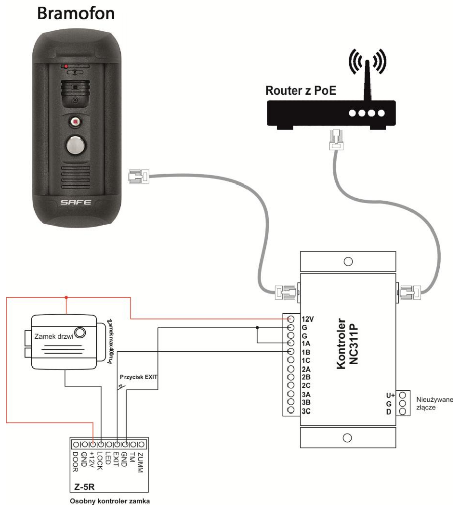
Rys. 4.9 (diagram poglądowy)
