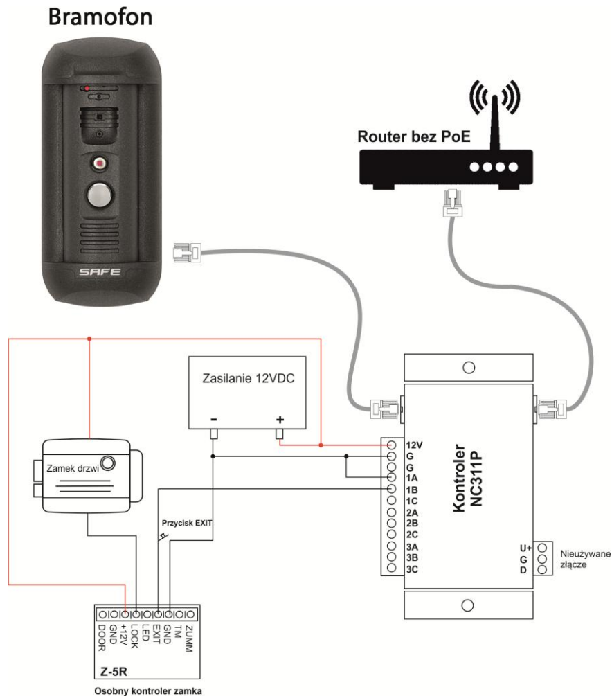
Rys. 4.7 (diagram poglądowy)
