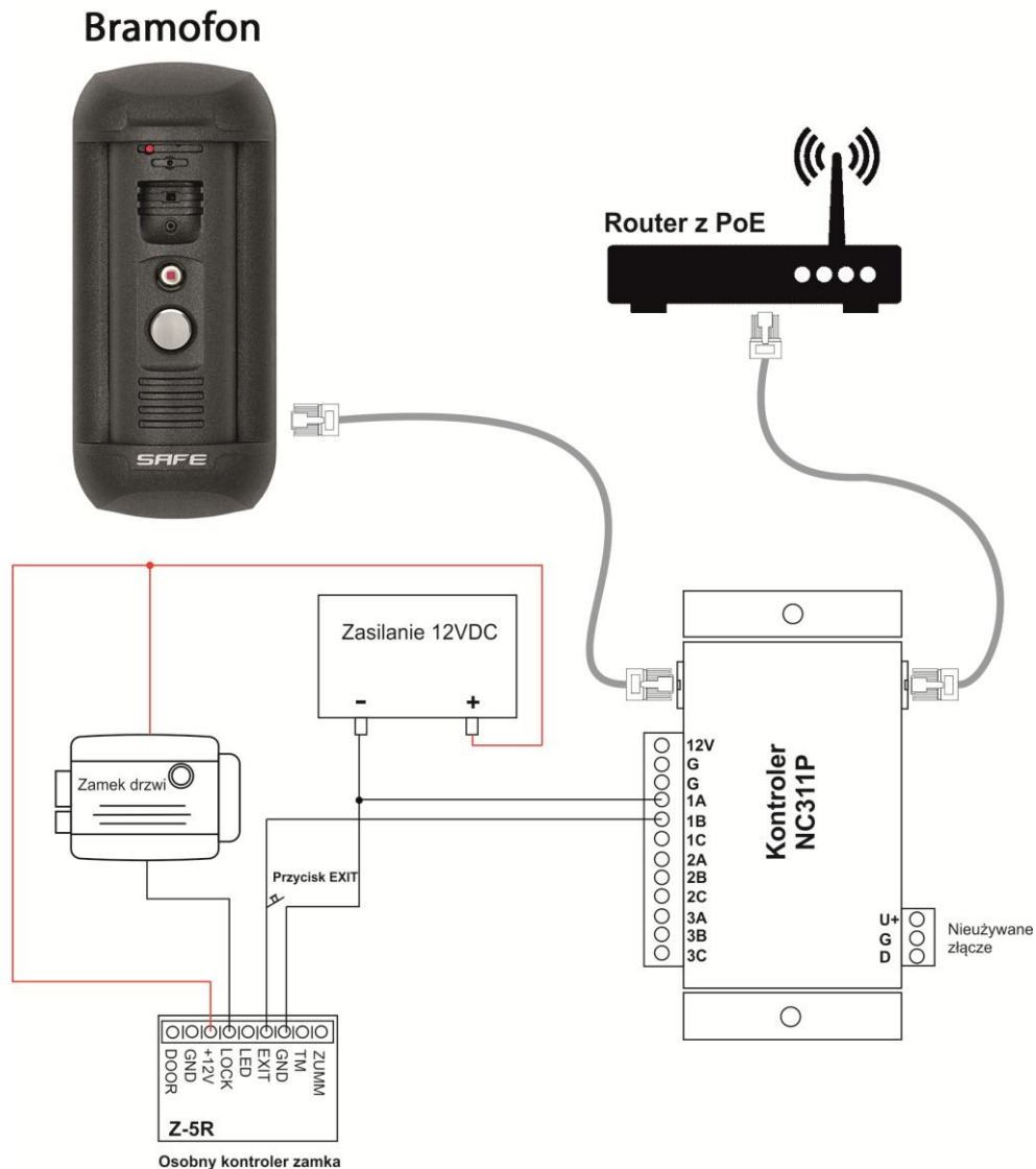
Rys. 4.8 (diagram poglądowy)
